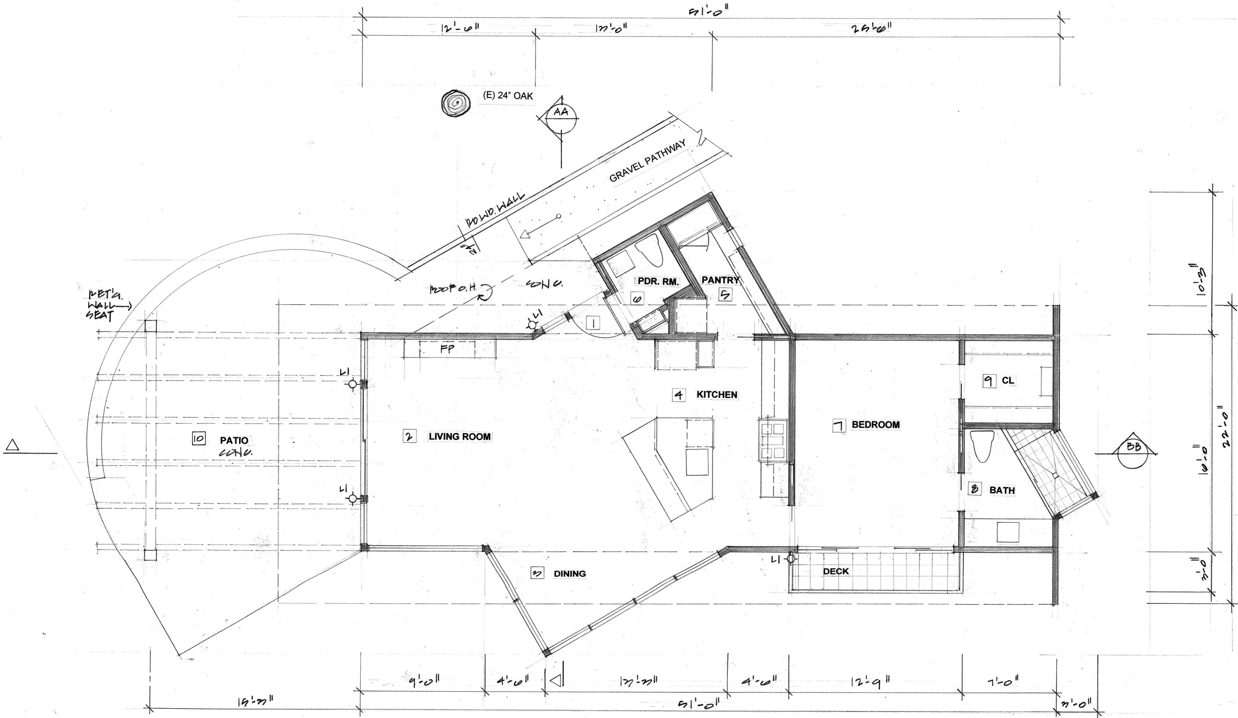
FLOORPLAN SCALE: 1/4"=1'-0"
